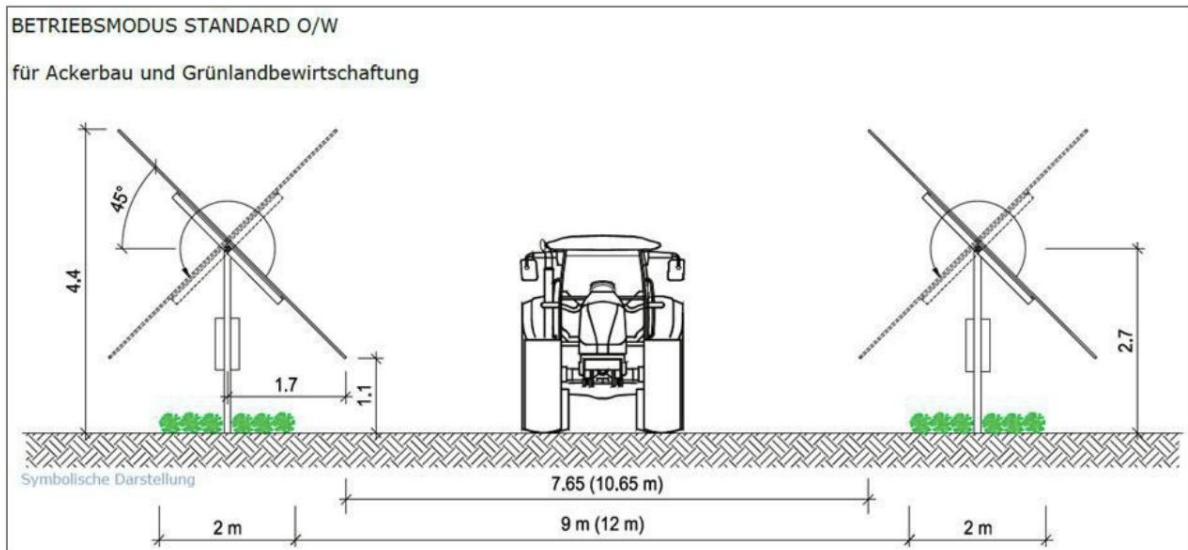
Abbildung 3: Skizze der Tracker
